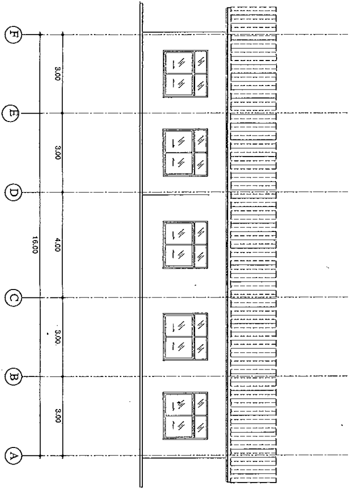
แบบรูปด้านหน้า มาตราส่วน 1:100
